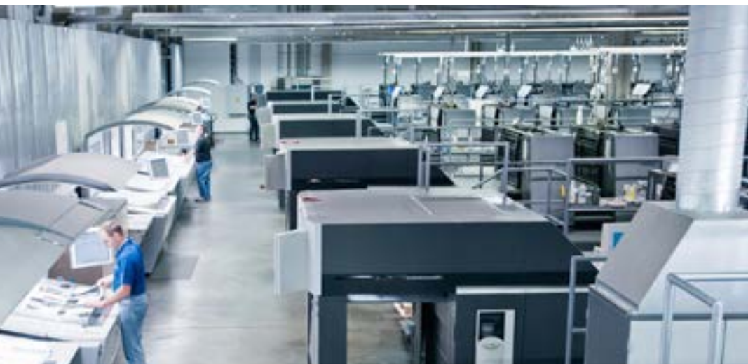
Bild 1 • Neue, hocheffiziente Pumpen sorgen für eine optimale Kühlung der Druckanlagen bei Aumüller. Bild: Aumüller Druck GmbH
